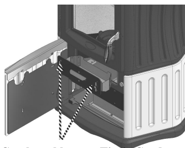
Crochets blocage- Tiroir Cendres
