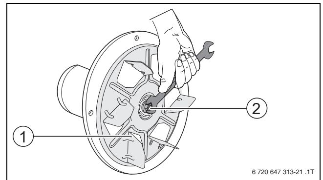
Obr. 9 Montáž oběžného kola ventilátoru
