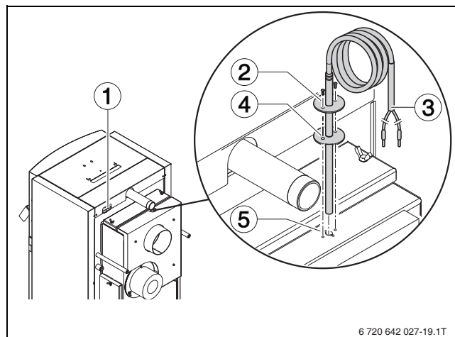
Obr. 12 Montáž čidla teploty spalin
