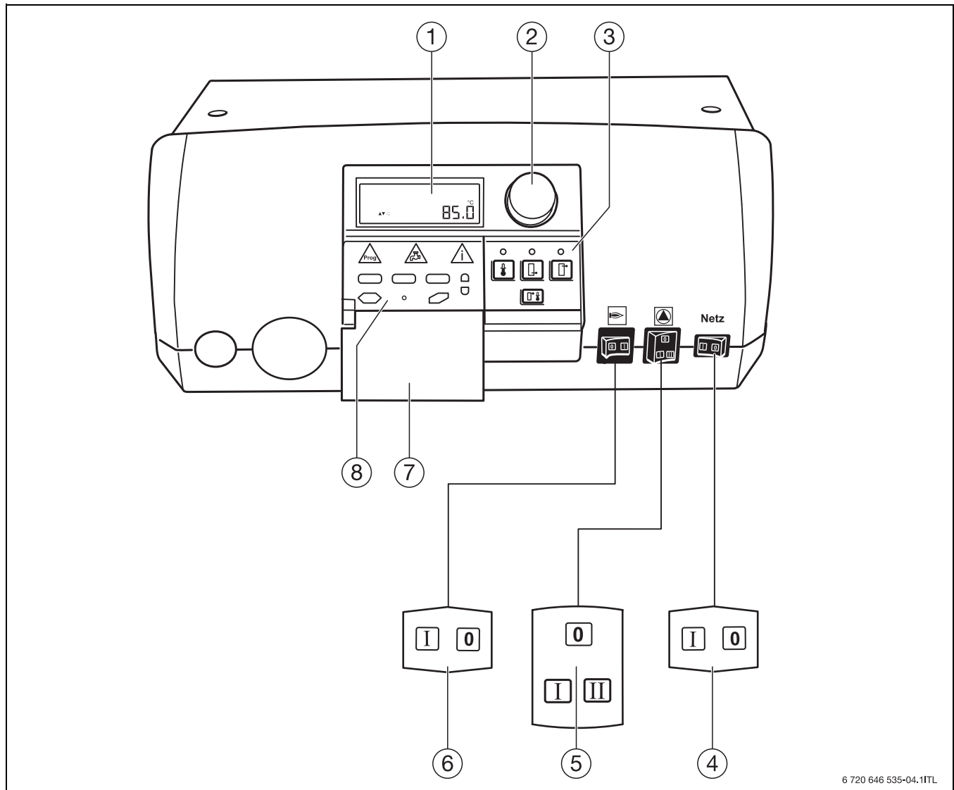
Obr. 31 Ovládací prvky regulačního přístroje
