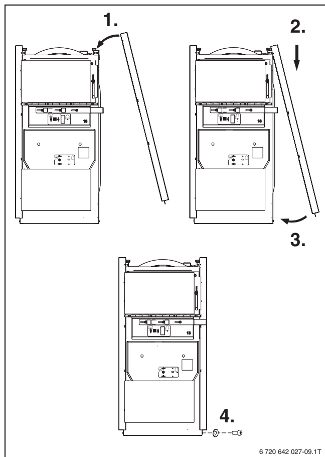
Obr. 16 Montáž bočního pláště
