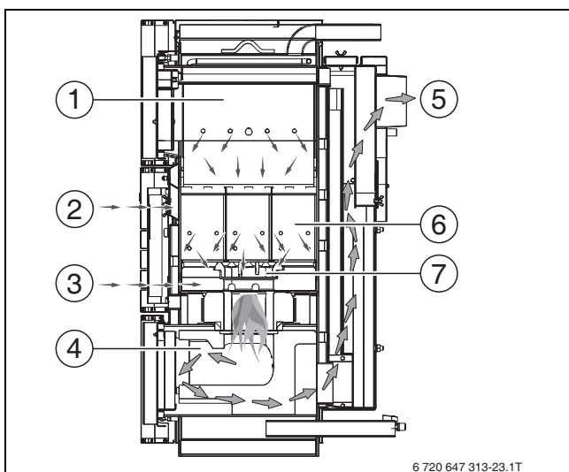
Obr. 38 Spalinová cesta
