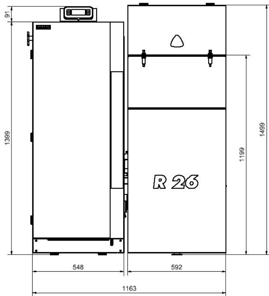
Obr. č. 5 Základní rozměry kotle BENEKOV R26
