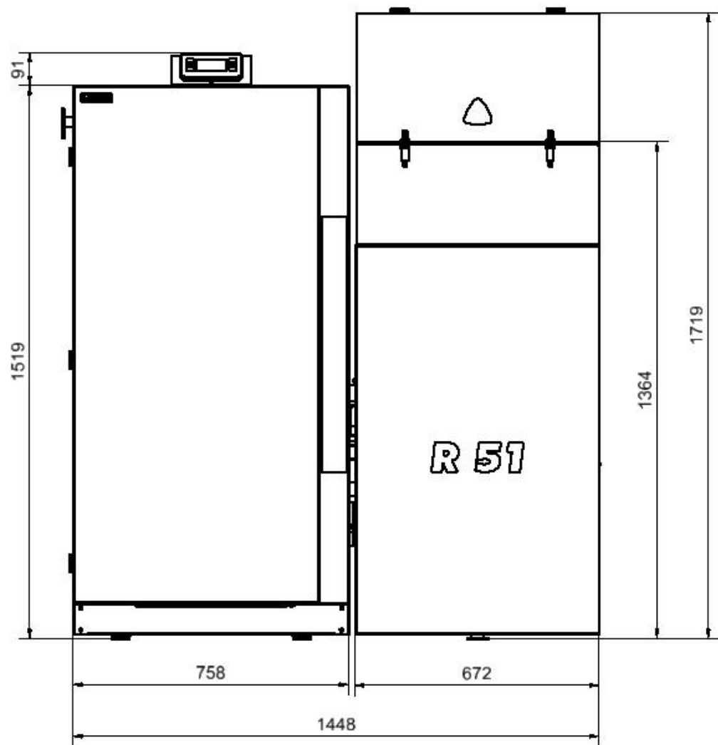
Obr. č. 6 Základní rozměry kotle BENEKOV R51
